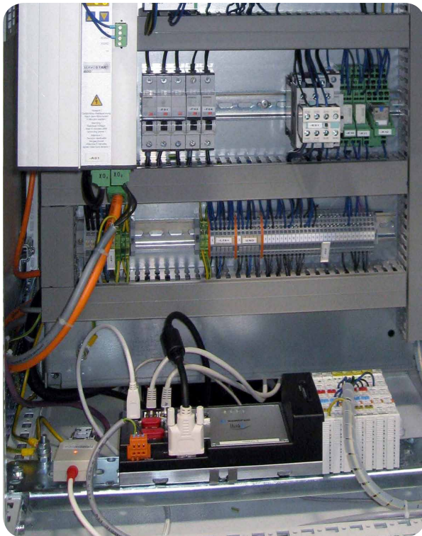
Bild 2 Der Kontron ThinkIO-Duo bietet ein umfangreiches Schnittstellenangebot, von Standard-PC- bis hin zu industriellen Feldbus- und Ethernet-Schnittstellen in einer einzigen, ultra kompakten Einheit.
